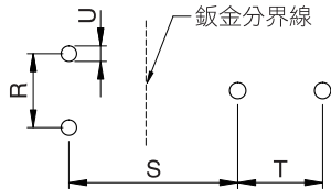
水平式安裝開孔尺寸
